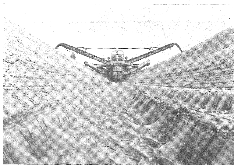
Tuksnesī rok guļni vienpadsmit kilometrus garam kanālam. Pa to ūdens no Ašhabadas Rietumu ūdenskrātuves atplūdis līdz zemju masīvam, kuru apgūst melioratori. Jāpiebilst, ka kanāla guļne būs betonēta.
