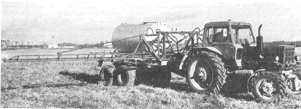
ATTEĻA: smidzināšanas iekārta uz organisko mēslojumu izkliedētāja ROU-6 bāzes.
