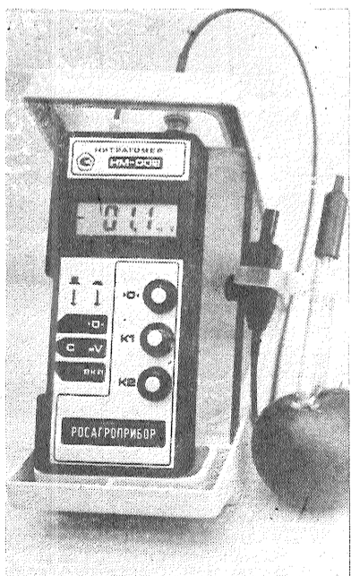
Portatīvais ekspresanalīzes aparāts «Mazulis NM-002», kura ražošanu sārijveidā nesēn uzsācusi specializētā rūpnieciskās projektēšanas un konstruktoru biroja «Ros-agropribor» eksperimentālā rūpnīca, paredzēts nitrātu koncentrācijas noteikšanai ūdenī, augsnē un lauksaimniecības produktos. Aparāta svārs ir apmēram 400 grami. Tā indikators parāda nitrātu koncentrāciju (mg) vienā svarā kilogramā vai vienā litrā šķidrums. Aparāta cena — 300 rubļu. Jauno aparātu varēs izmantot agronomi un ārsti, bērnu darza un skolu pavāri, dārzu sagādnieki. ATTEĻA: nitrātu koncentrācijas mērītājs aparāts «Mazulis NM-002».
