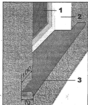
1 – logs. 2 – loga aile. 3 – koka palodze. Koka palodze ar pārlaidumu – palodze izvērta 70 mm uz āru un galos 100 mm pārlaidumi.
