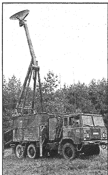
● Novērošanas radars PS-70, kas ir paredzēts gaisa telpas novērošanai un mērķa datu nosūtīšanai uz uguns vienībām (RBS-70). Apkalpe strādā četri karavīri, darbības rādīss ir 20 vai 40 km un izvēršanas laiks ir 15 minūtes.
