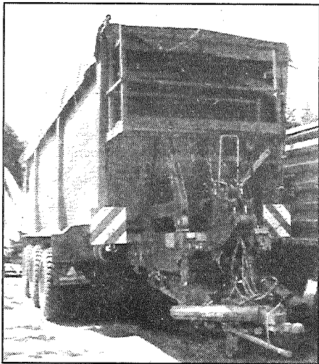
● Baltijā lielākā piekabe ar celtspēju 33 tonnas.
