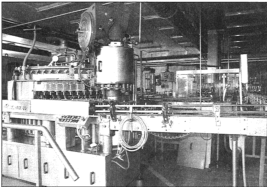
● Attēlā redzama alus pildīšanas iekārta. Te stikla pudelēs iepilda dzērienu.
