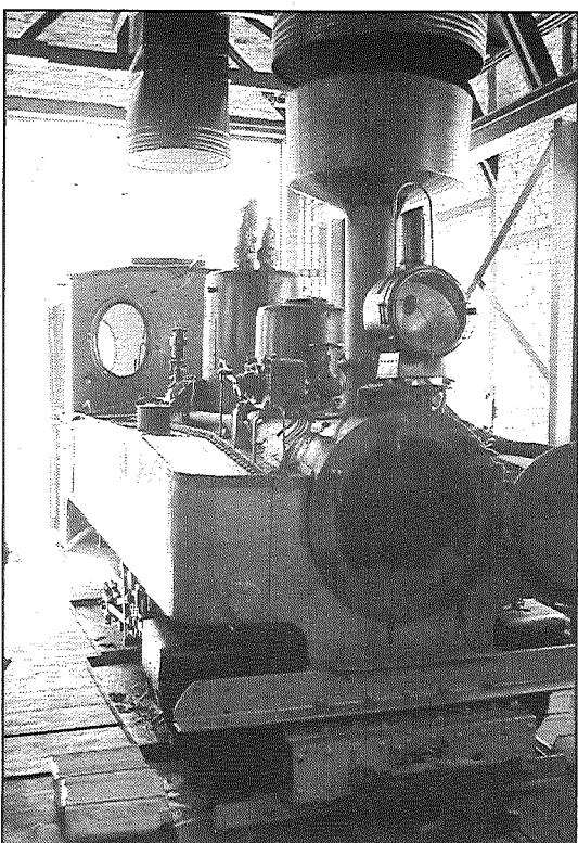
● Tāda izskatās bāniņa lokomotive, kuras tvaika katls savās jaunības dienās sasniedza 12 atmosfēru spiedienu, nu vairs tikai vidēji 6,5 līdz septiņas atmosfēras.
