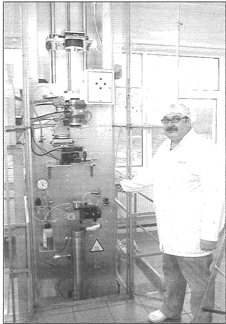
● Gaismas vada vilkšanas procesa sākums šķiedras vilkšanas tornī. Optiskā šķiedra tiek vilkta no kvarca stikla formām temperatūrā no plus 2000 līdz 2100 grādiem. Tehnoloģisko procesu žurnālistiem skaidro optisko šķiedru vilkšanas iecirkņa vadītājs Jānis Škapars. Foto: A. Šņepsts
