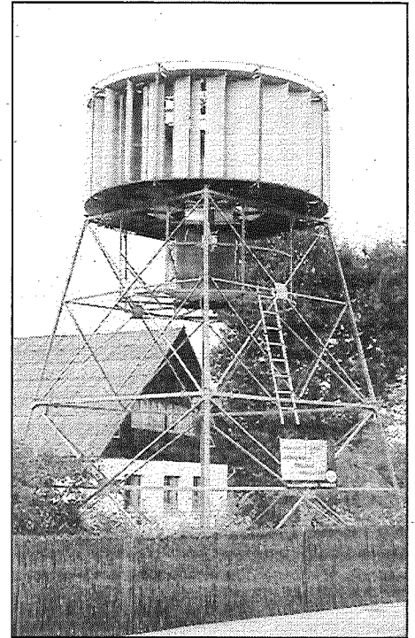
● Vēja ģenerators.
