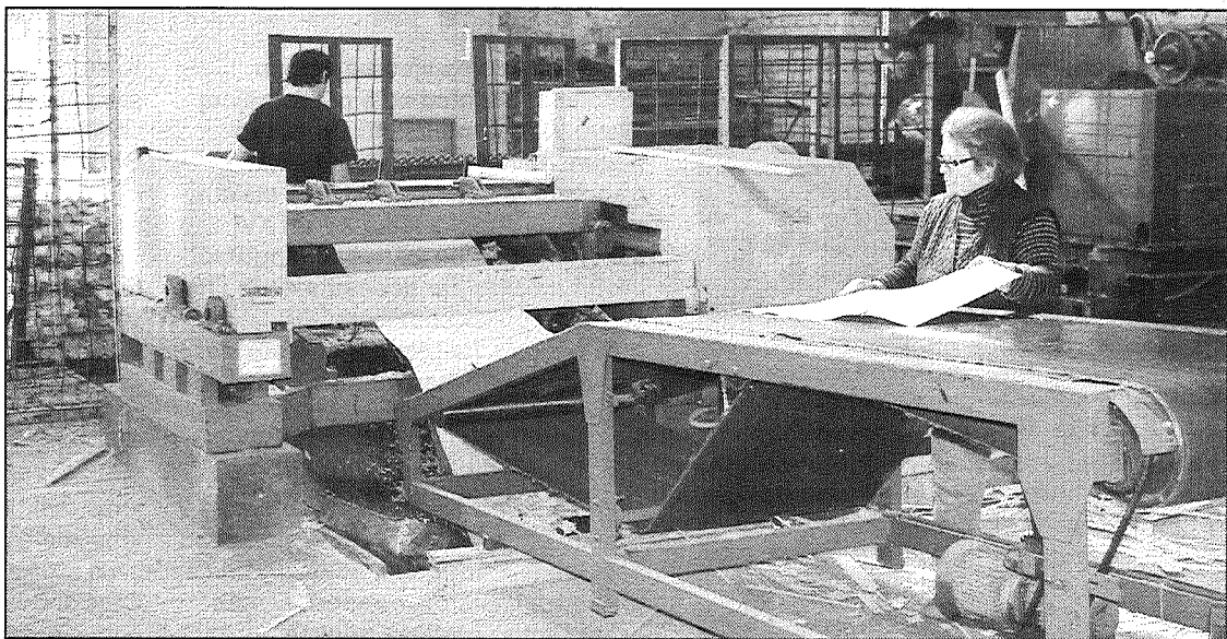
● Lobīto taras dēļišu ražotnē SIA “Aglonas serviss” ražošanas process ir pilnībā automatizēts. Viena no iekārtām apses klučus loba plāksnēs, no kurām tālāk tiks gatavotas kastīšu pamatnes.
