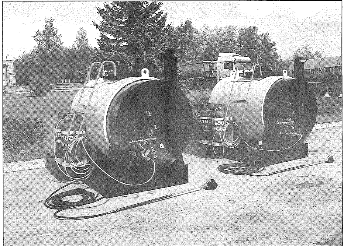
● Tā izskatās preiļiešu izgatavotā iekārta asfaltbetona segas bedrīšu remontam ar bitumena emulsiju.
